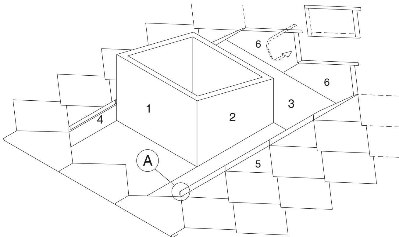
DETTAGLIO "A" aperto
